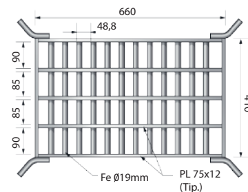
Sumidero tipo S2
