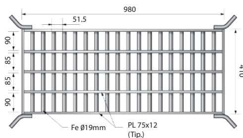
Sumidero tipo S1
